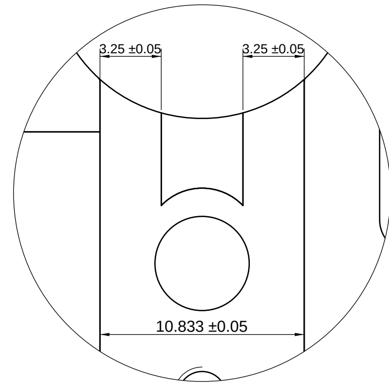
A (5 : 1)
